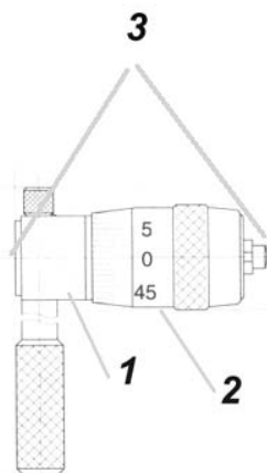
Rod Type Internal Micrometer Rute Inneres Mikrometer Il Tipo di verga Micrometro Interno
